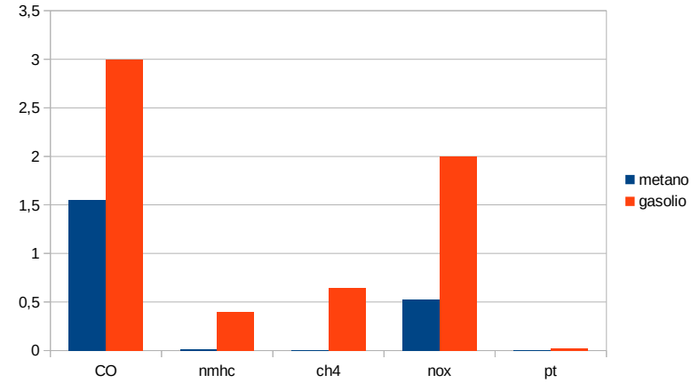
EMISSIONI GAS DI SCARICO PER KW/h
